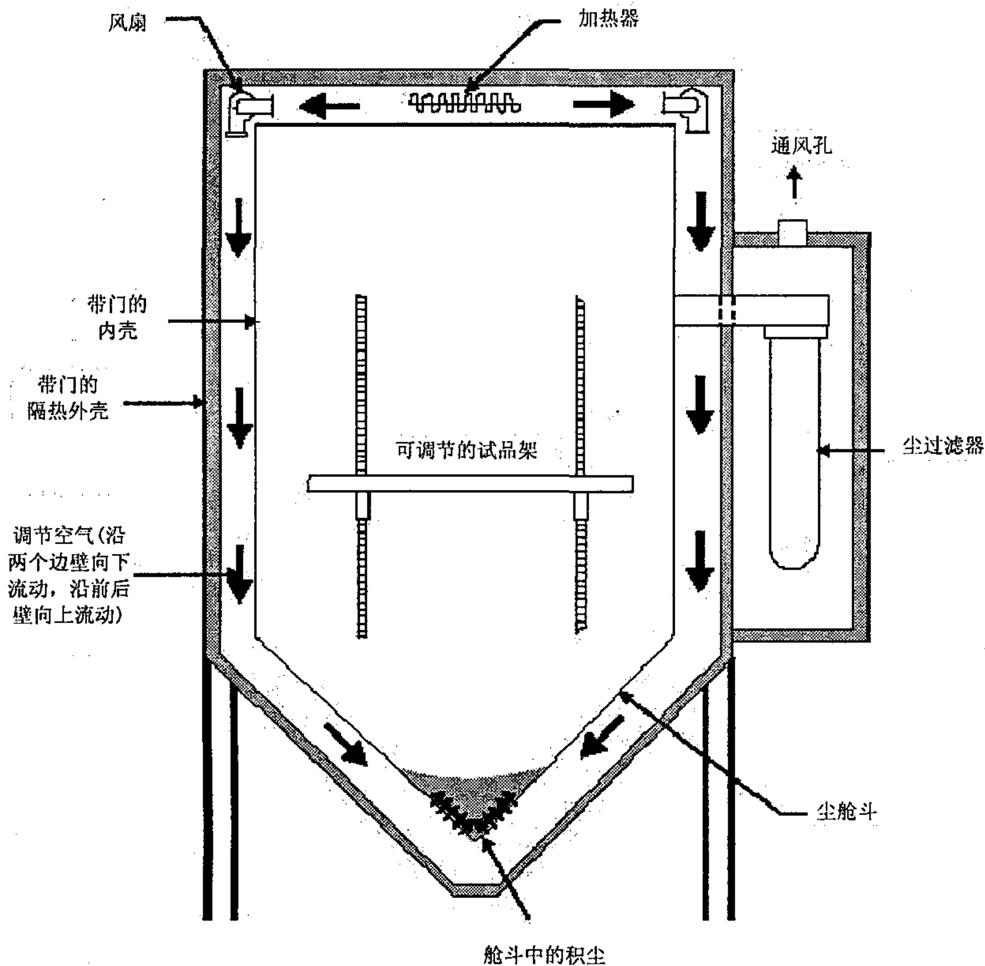
图1 降尘试验装置示例
