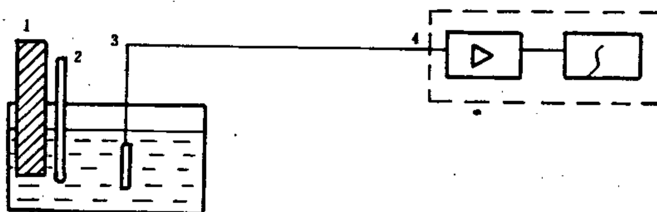
图 3 浸提式恒温水槽温度波动度的测试
